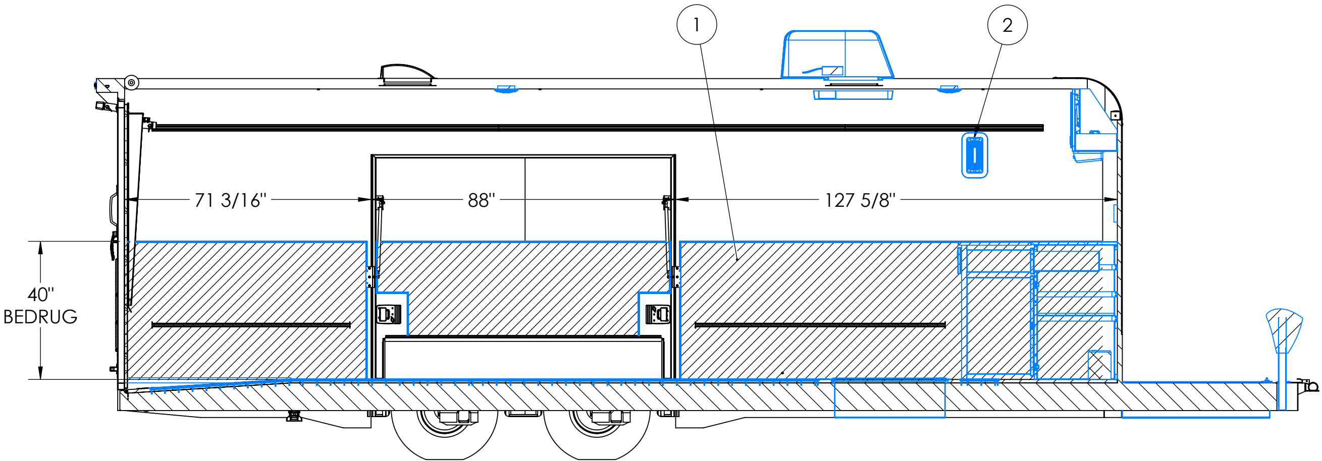
SECTION D-D SCALE 1 : 28
